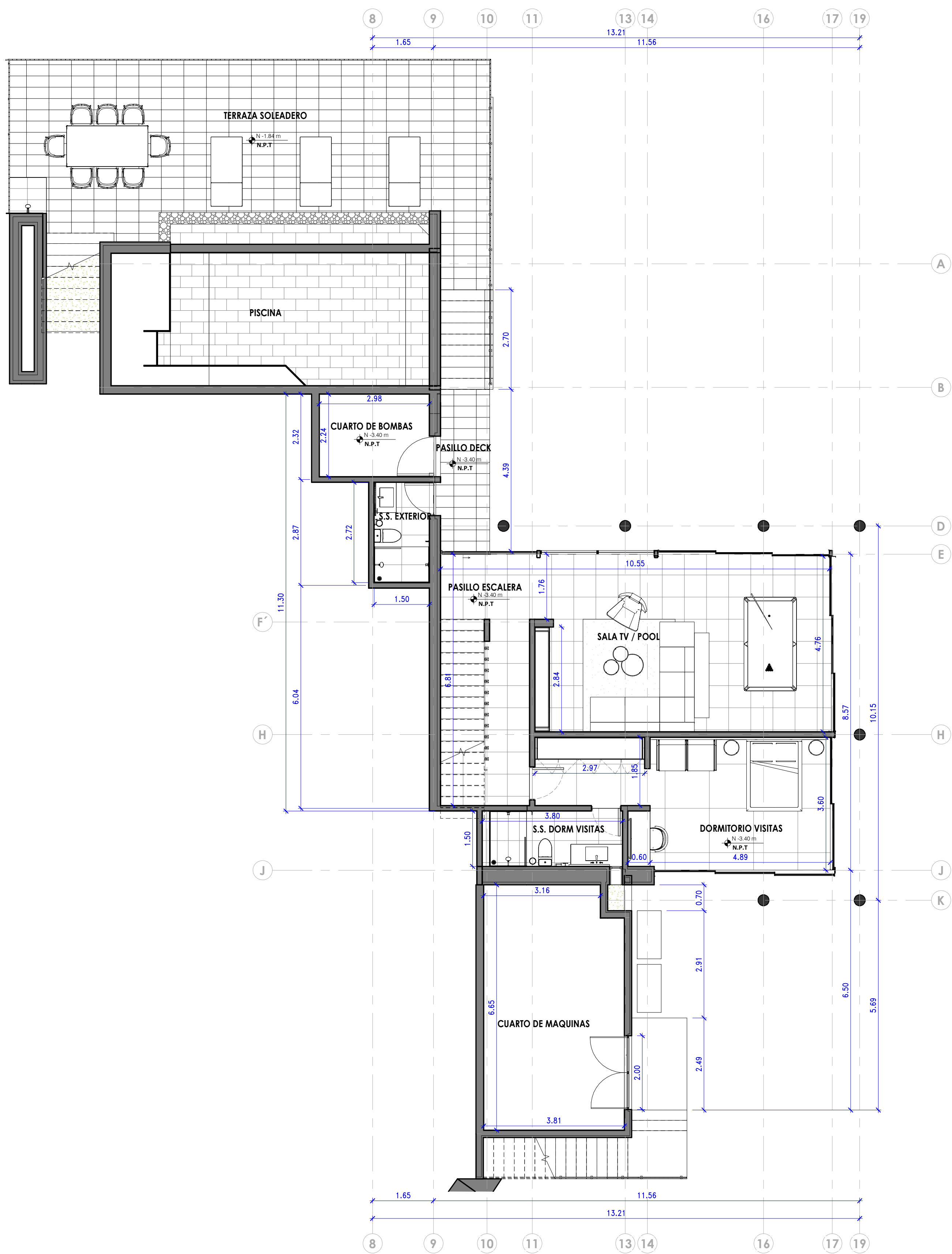
2 PLANTA ARQUITECTONICA NIVEL S100 ESCALA: 1 : 75
