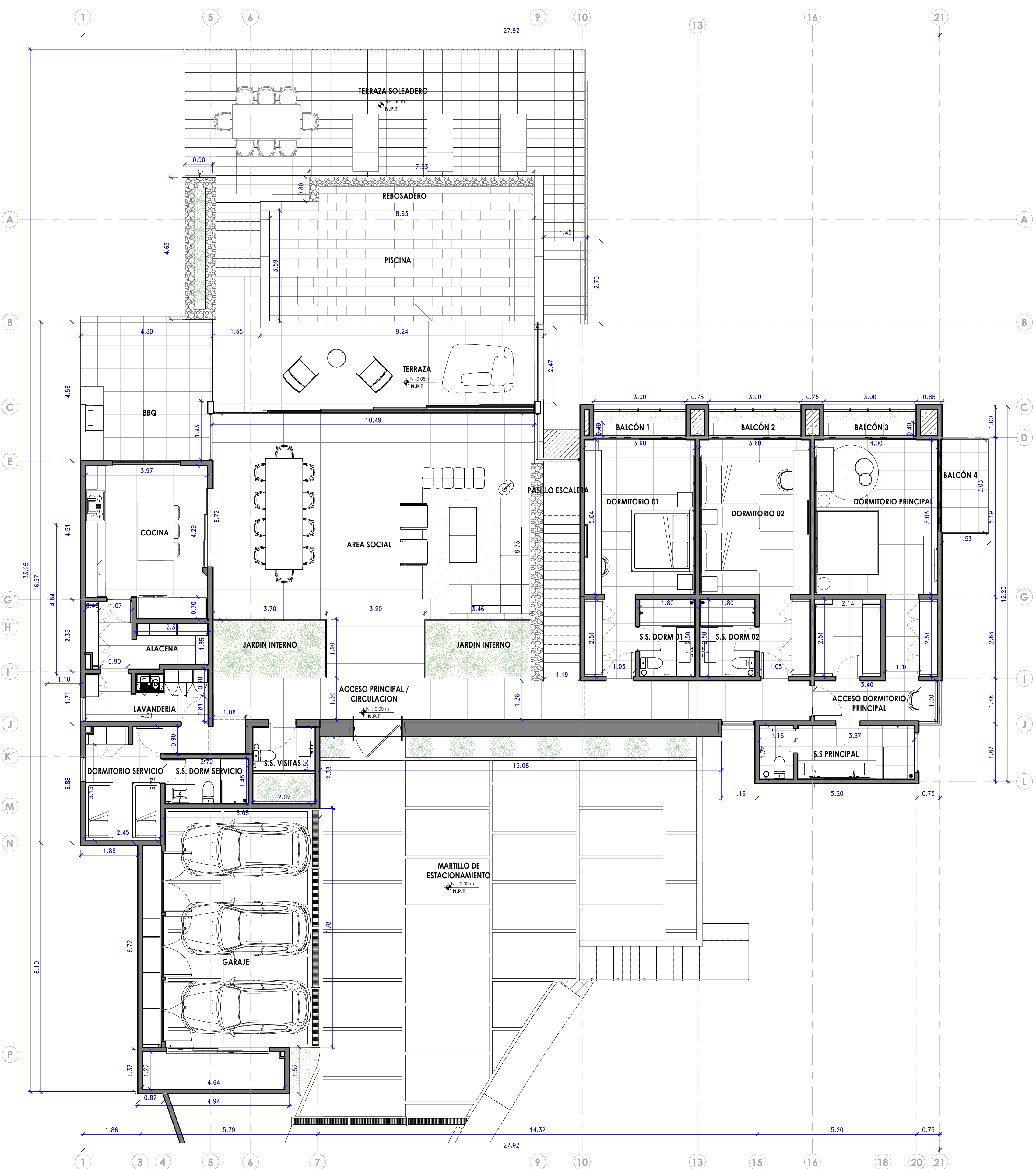
1 PLANTA ARQUITECTONICA NIVEL N100-PRESENTACIÓN ESCALA: 1 : 75
